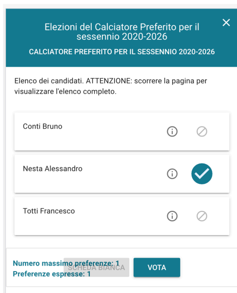
Figura 9: Candidato selezionato
