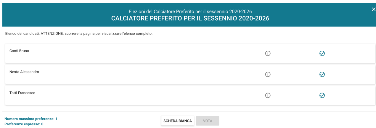
Figura 4: Elenco Candidati.
