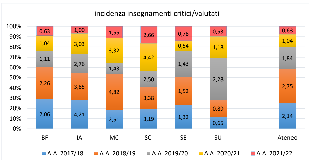
FIGURA 1 - DISTRIBUZIONE INCIDENZA PERCENTUALE DEGLI INSEGNAMENTI CRITICI SUI VALUTATI, PER FACOLTÀ.
